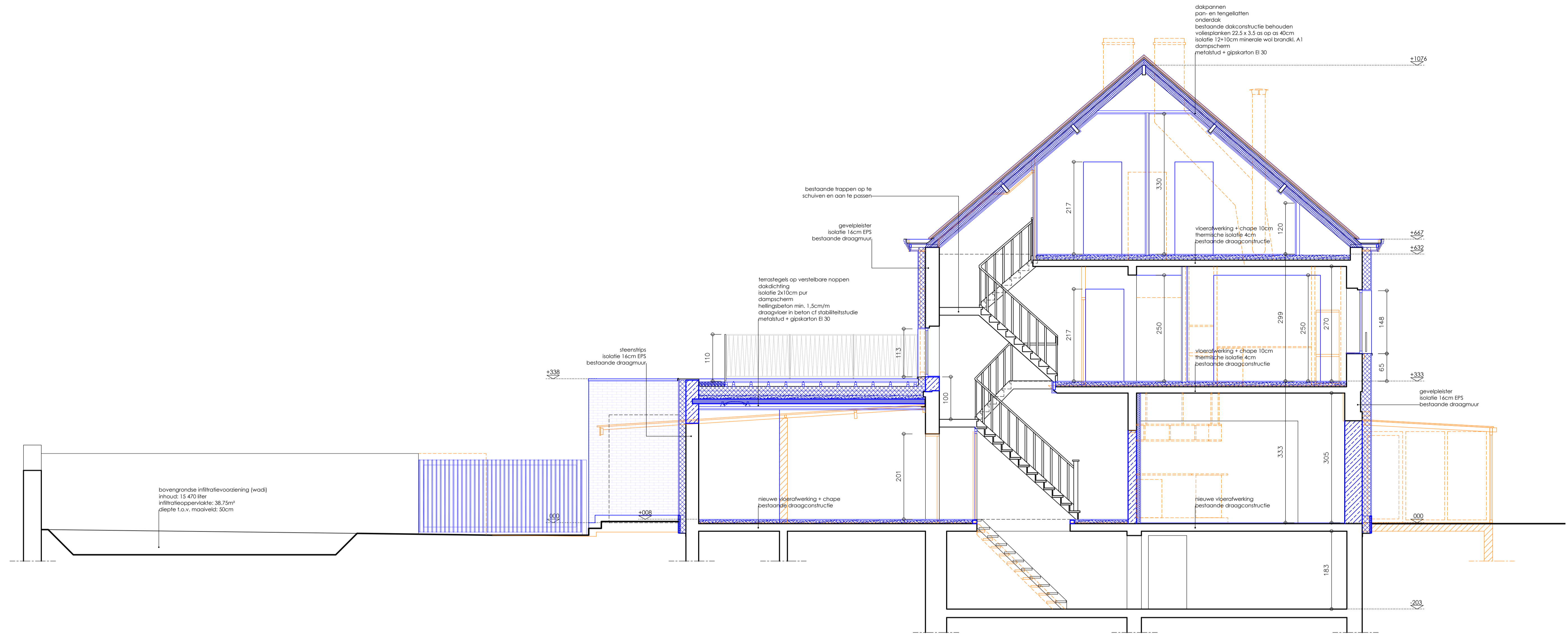
DOORSNEDE BB
