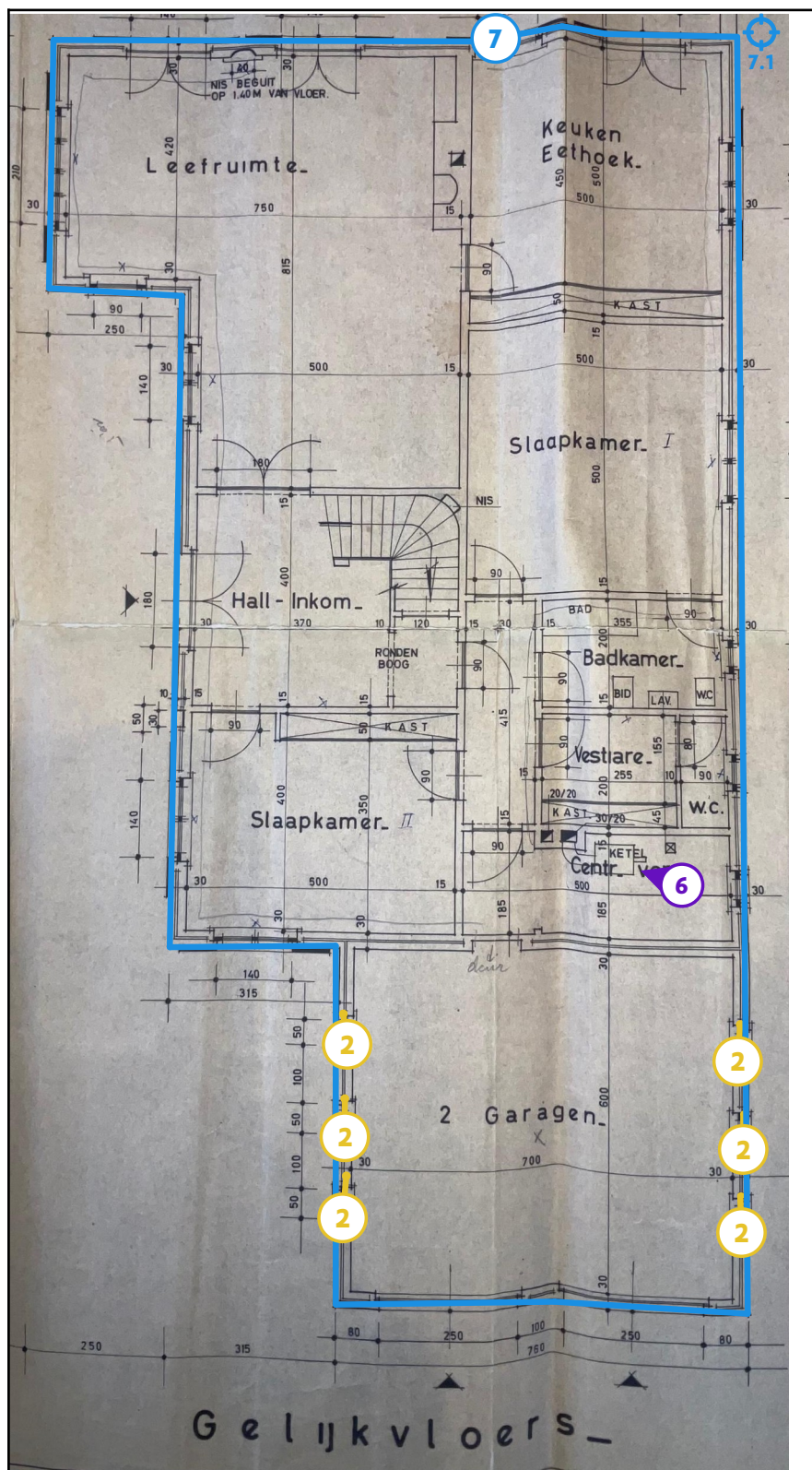
Legende van plan 1.1: Gelijkvloers - massal - cv - crepi
