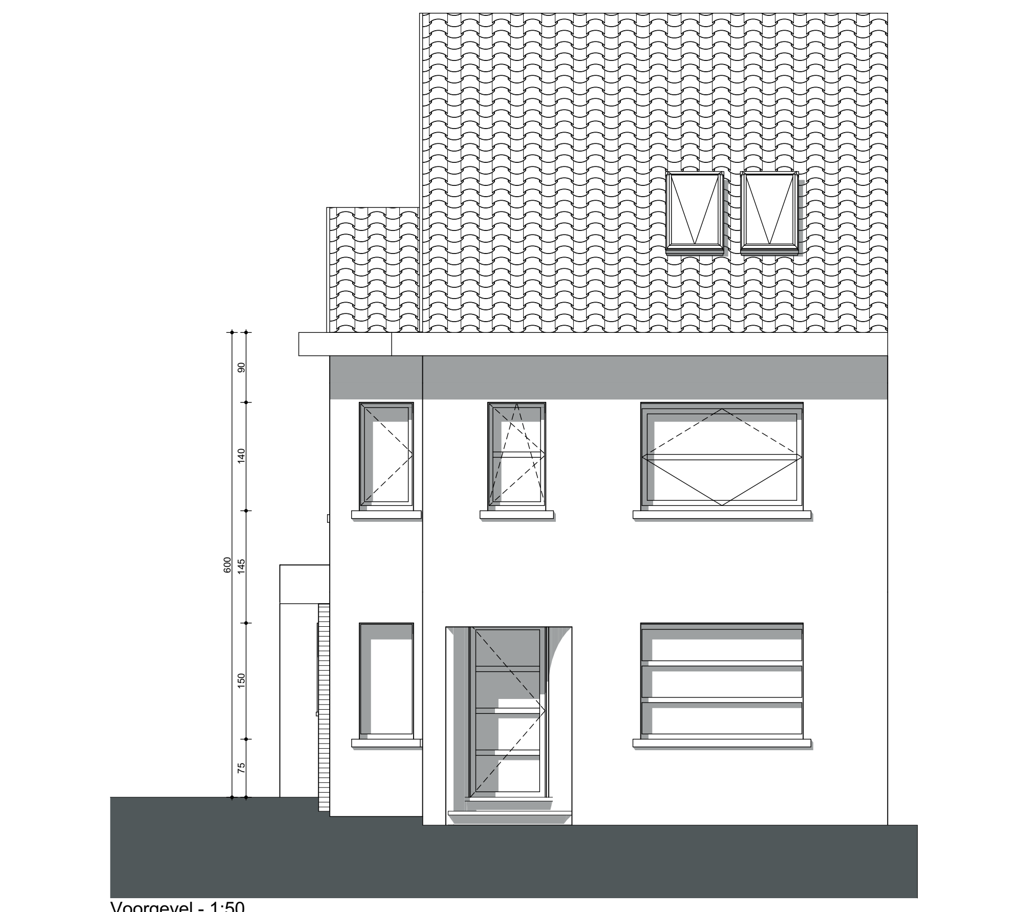
Voorgevel - 1:50
