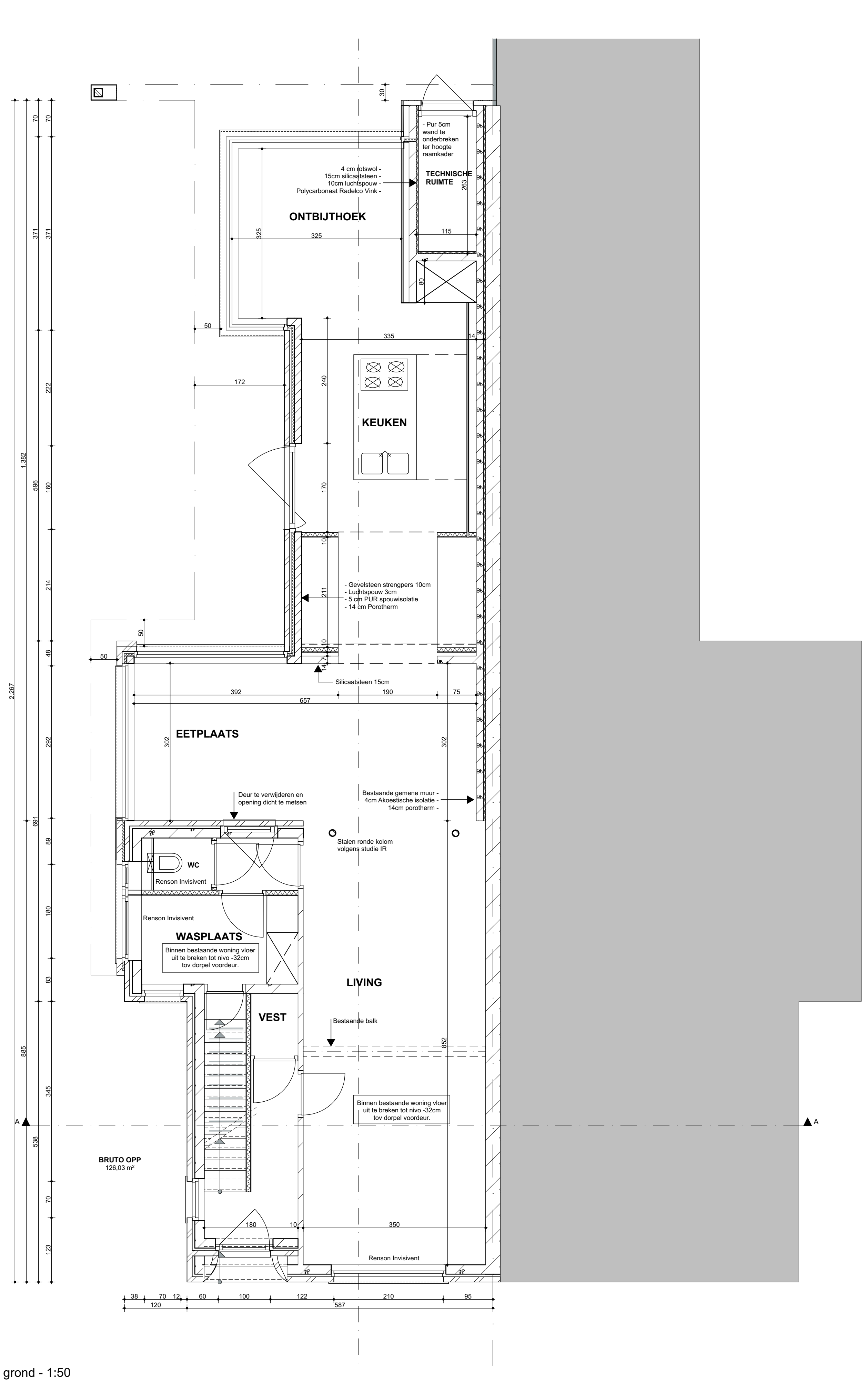
Begane grond - 1:50
