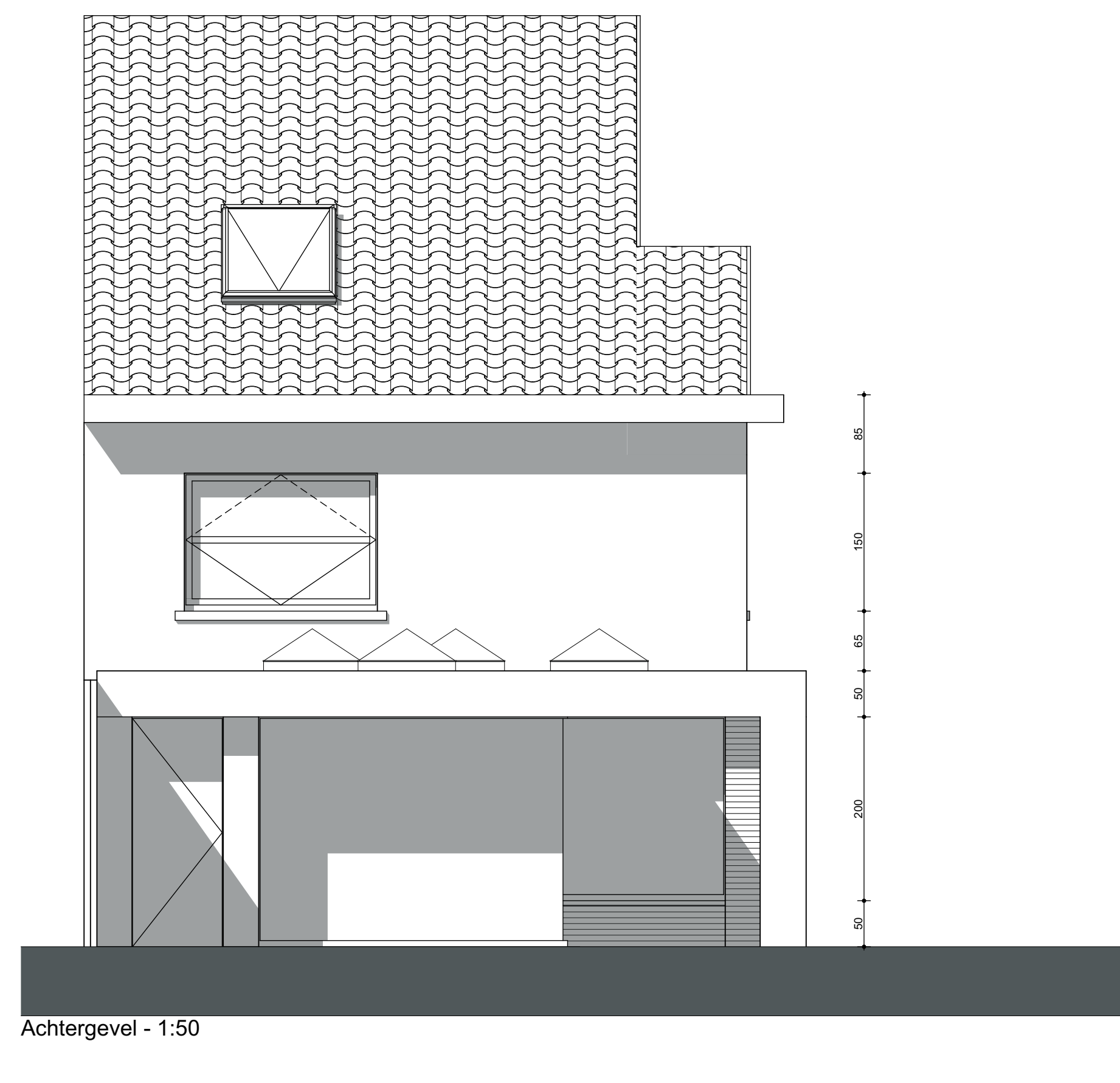
Achtergevel - 1:50
