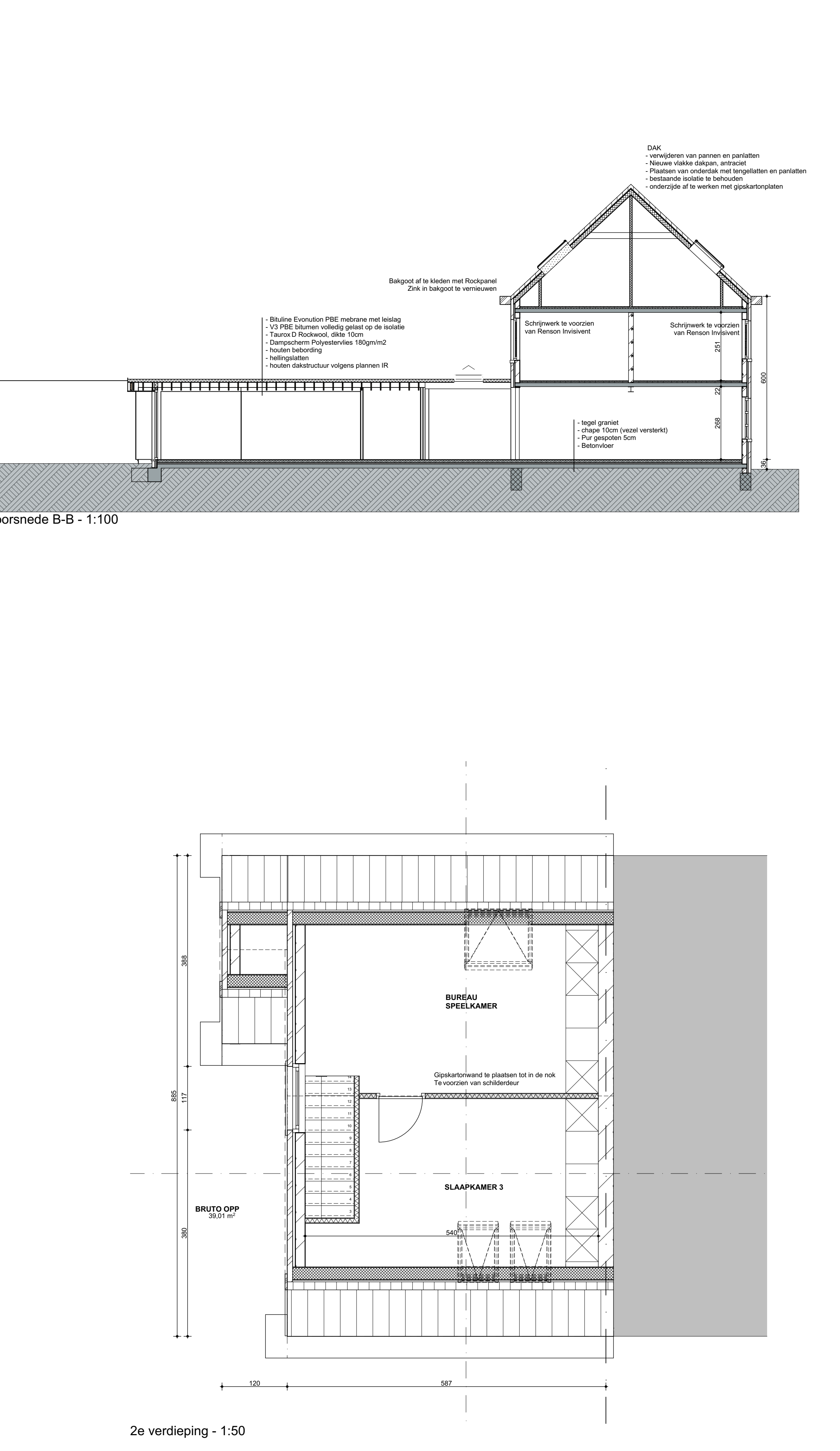
2e verdieping - 1:50
