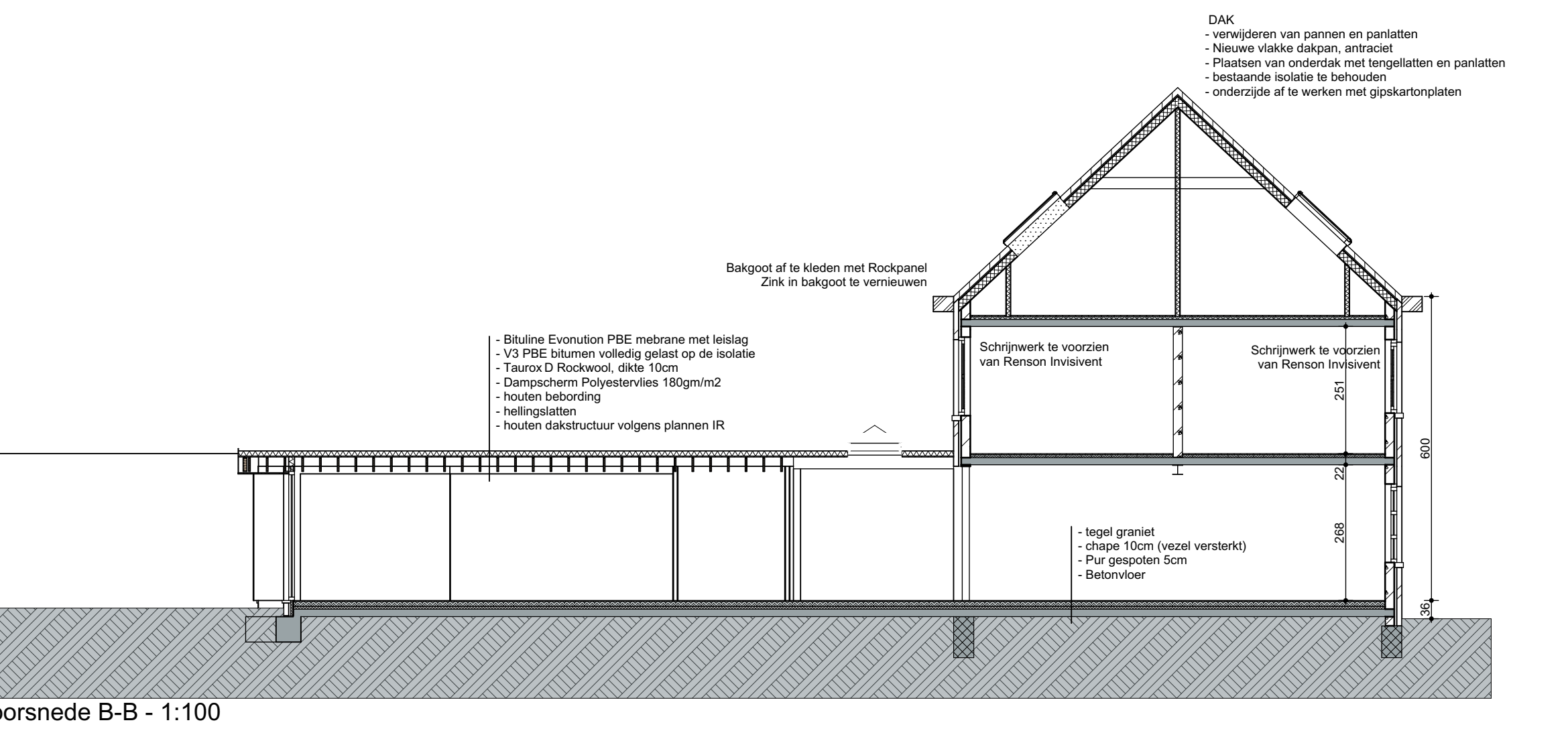
Doorsnede B-B - 1:100
