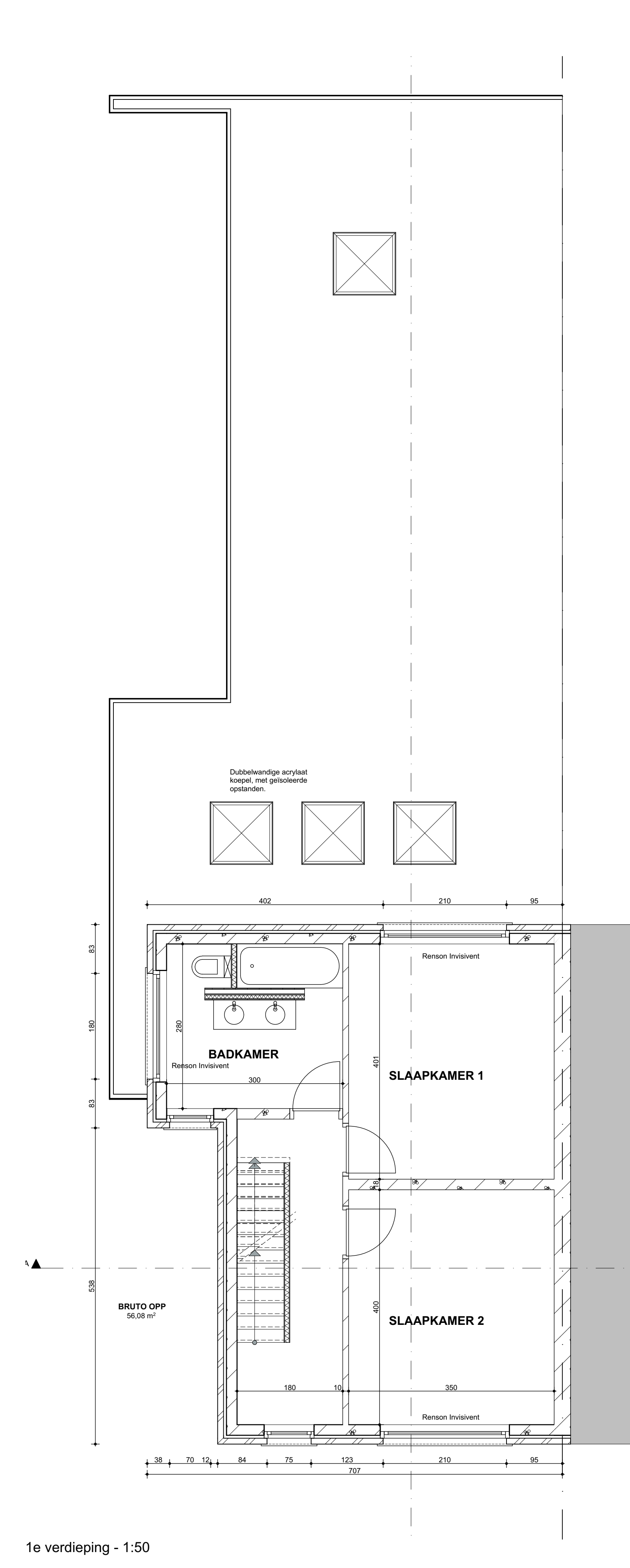
1e verdieping - 1:50
