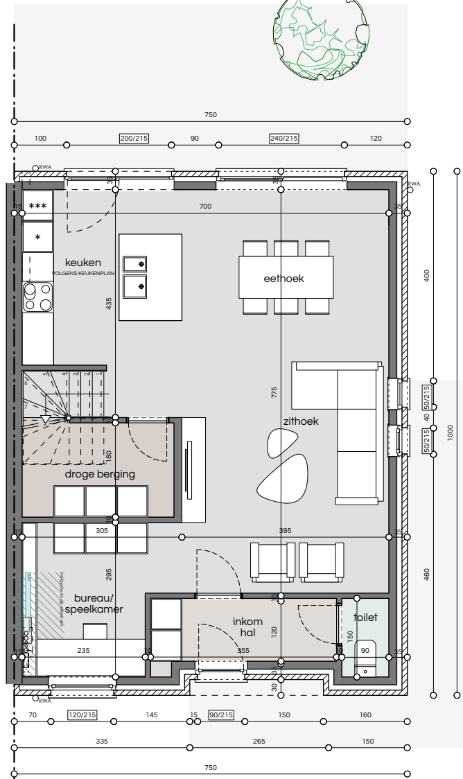
GRONDPLAN gelijkvloers
